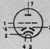
Miniatur B7G
